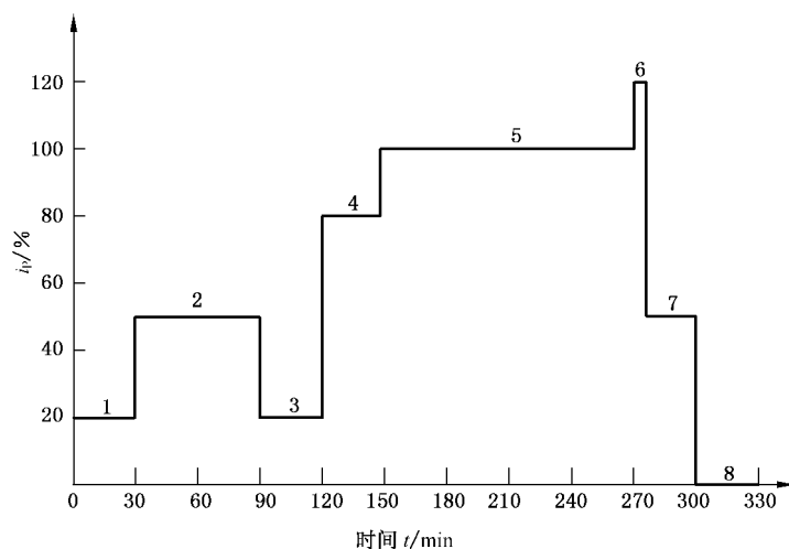
图 2 试验循环工况曲线
